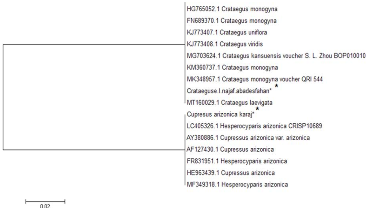
▲ نمودار ۲-رسم درخت فیلوژنی بر اساس ساختار doohilekil mumixam صورت گرفته است. این درخت بر اساس ناحیه lcb در هر دو گونه سرو نقره‌ای و زالزالک در یک تست رسم شده است. همان‌طور که در تصویر مشخص است به خوبی دو گونه از هم تفکیک شده اند. دو گونه ستاره دار شده نمونه‌های مورد مطالعه در این پژوهش هستند.
