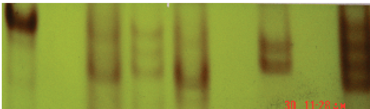
LPL کنترل منفی کنترل مثبت Ph-Ch GuSCN Ph-Ch GuSCN نمونه ۱۵ نمونه ۹ نمونه ۲
